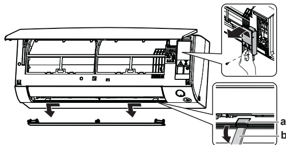
a Завинтващ се капак b ооо символ
