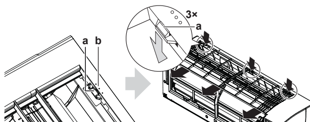
a Горна кука b ооо символ
