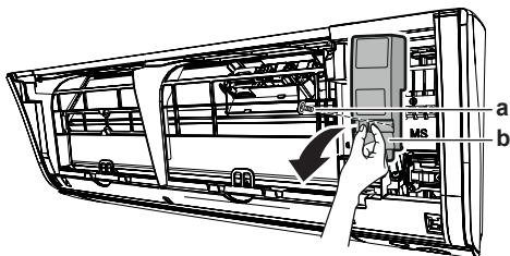
a Винт на сервисен капак b Сервисен капак
