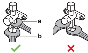
a Гаечен ключ b Динамометричен гаечен ключ
