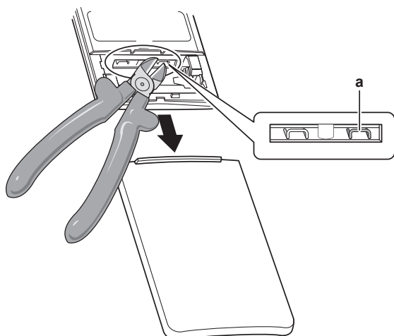
а Адресен джъмпер J4
