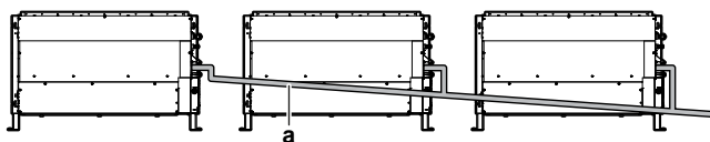
a Централна дренажна тръба (с наклон от поне 1/100)
