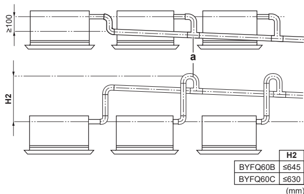
a Т-съединение
