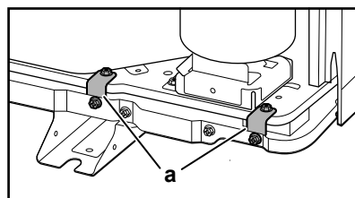
a Транспортни подложки (2x)
