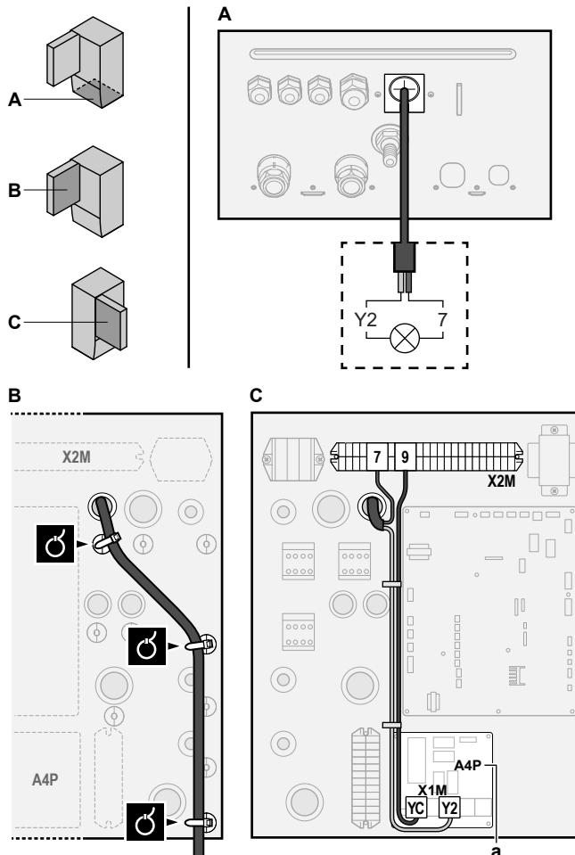
a Изисква се монтаж на EKRП1НВАА.
