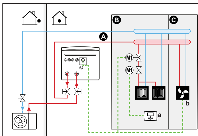
A Основна зона на температурата на изходящата вода
