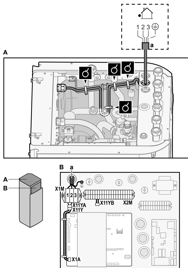
a Соединителен кабел (=главно електрозахранване)
