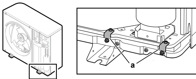
a Транспортни подложки (2x)
