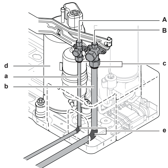
A Спирателен клапан (течност) B Спирателен клапан (газ) a Тръбопровод за течност b Тръбопровод за газ c Изолационни краища d Компресор e Винилова лента
