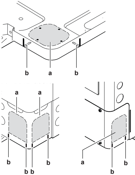
a Пробит отвор за тръбопровод b Прорез
