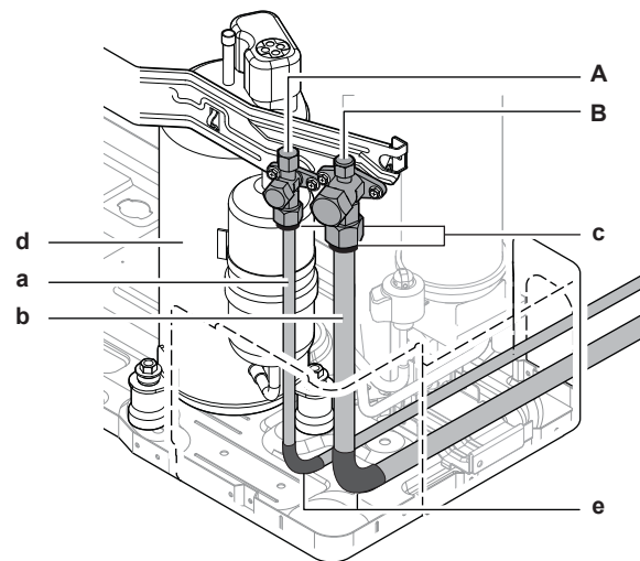
A Спирателен клапан (течност) B Спирателен клапан (газ) a Тръбопровод за течност b Тръбопровод за газ c Изолационни краища d Компресор e Винилова лента
