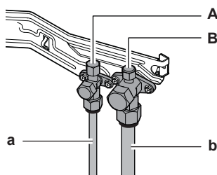
A Спирателен клапан (течност) B Спирателен клапан (газ) a Тръбопровод за течност b Тръбопровод за газ
