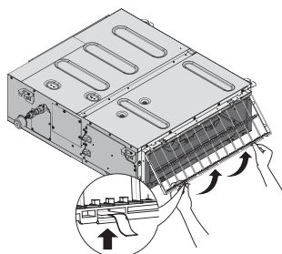
задно всмукване
